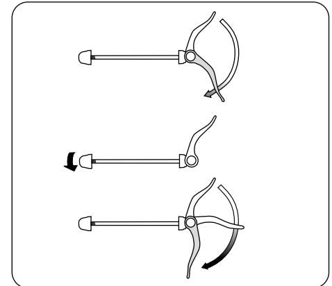
Einstellmutter anziehen
