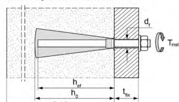
Ankerstange im konischen Bohrloch
