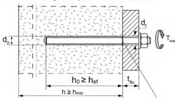
Ankerstange im zylindrischen Bohrloch
