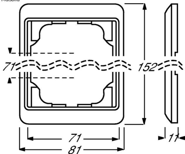
Maßbild
