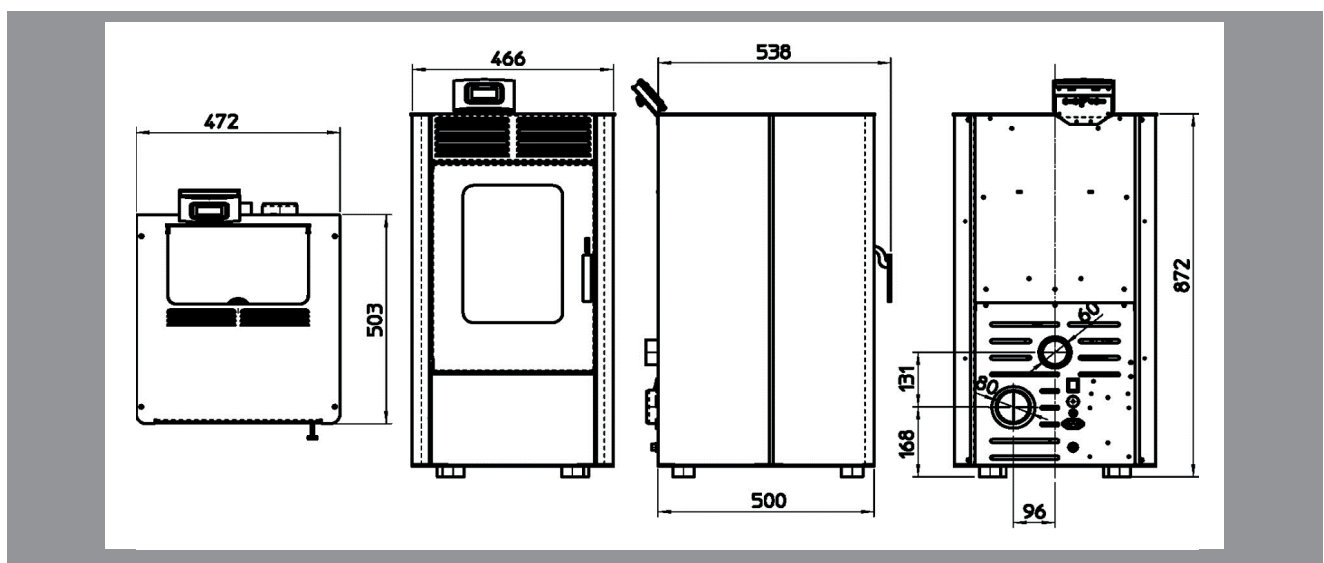
Abb. 1b: Geräteabmessungen (alle Maßangaben in mm)
