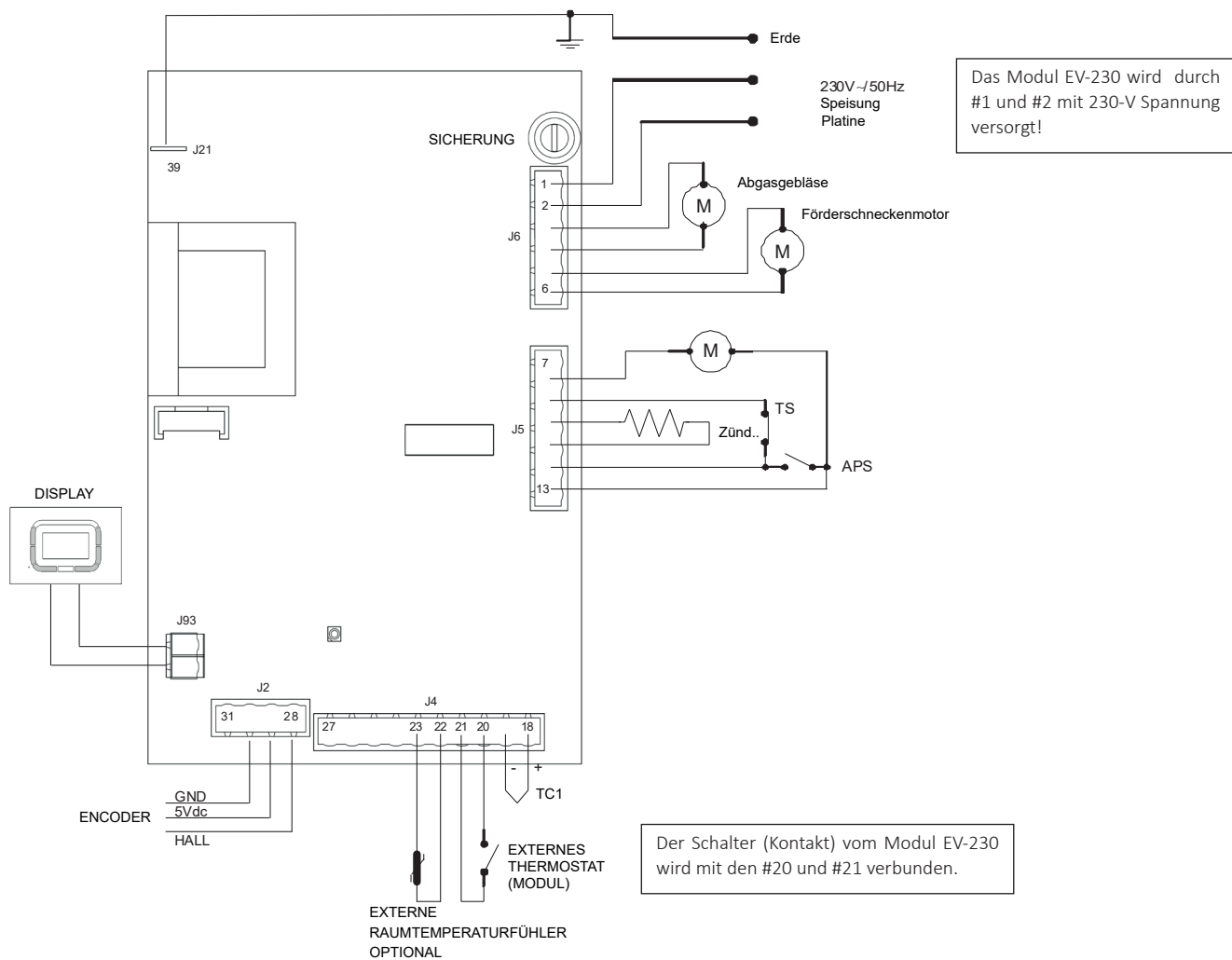
Abb. 15: Schaltplan der Platine
