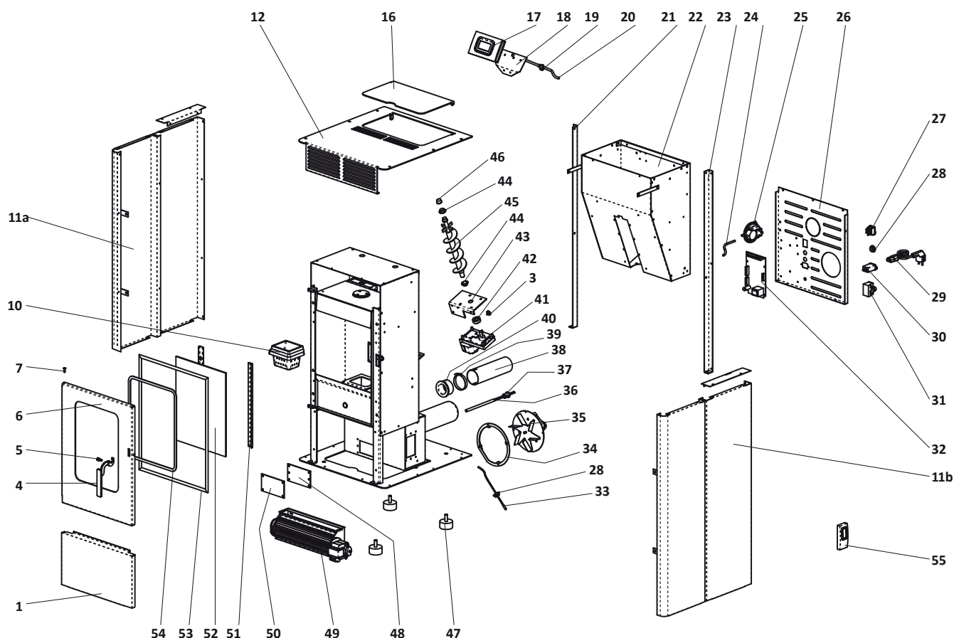
Abb. 14 Explosionszeichnung
