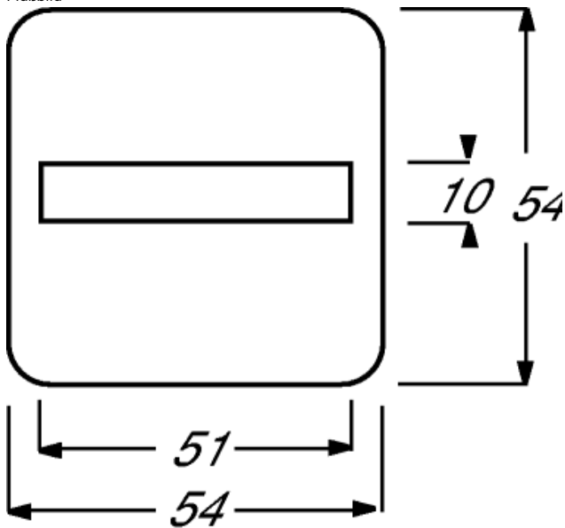
Maßbild
