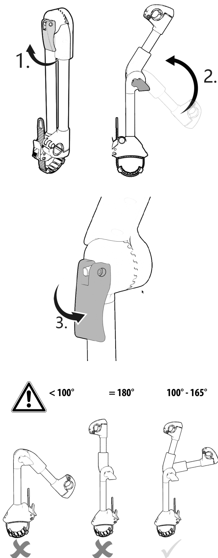
Figura 2: Ribaltamento del supporto del telaio
