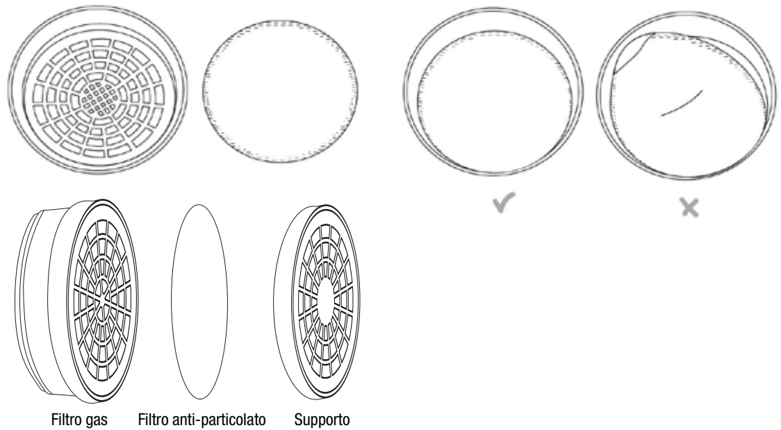
Filtro gas Filtro anti-particolato Supporto
