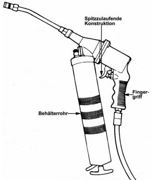
Abb.1: Druckluft-Fettpresse
