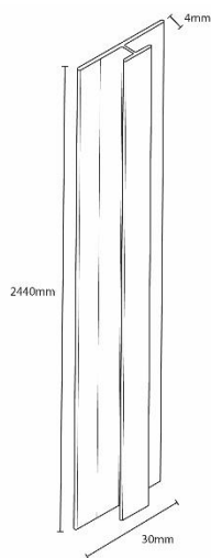
H-Verbindung
