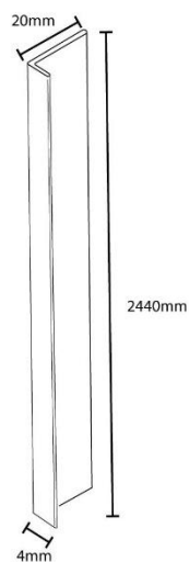
Endkappe
