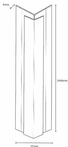
Außenecke
