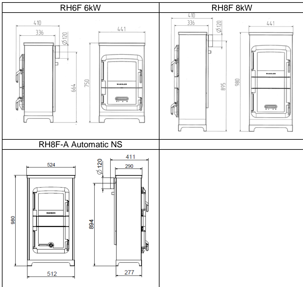
Fig. 3.: RH8F-A Automatic NS 8kW
