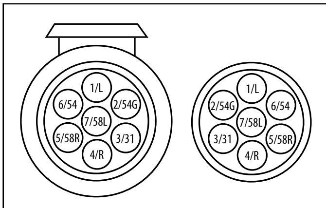
Bild 25: 7-poliger Elektroanschluss
