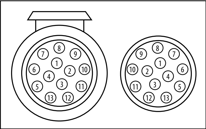
Figure 2 : Raccordement électrique à 13 broches
