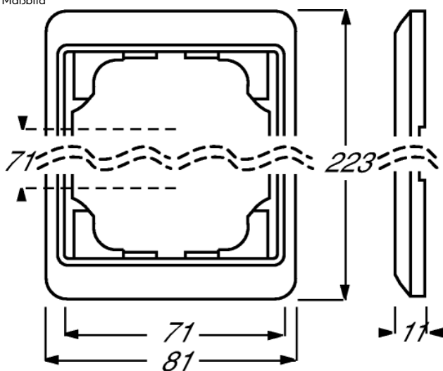
Maßbild
