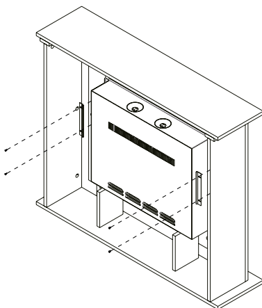
VERWENDEN SIE 4 SCHRAUBEN DES TYPST 3,5 X 12
