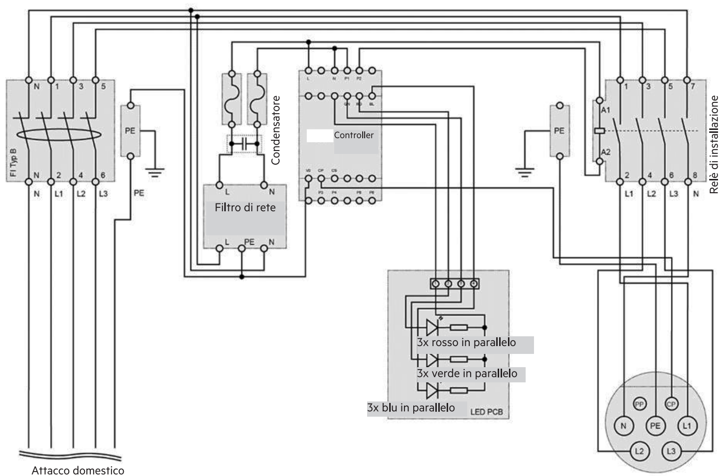
Fig. 5: Schema elettrico 11202, 11204
