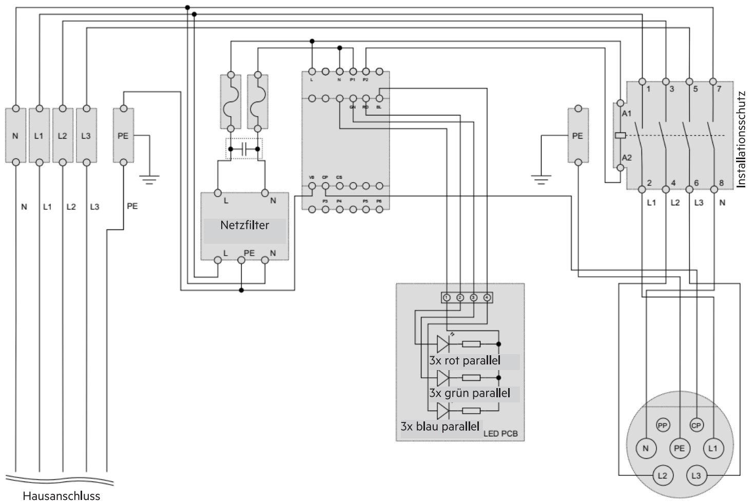
Abb. 4: Schaltplan 11201, 11203
