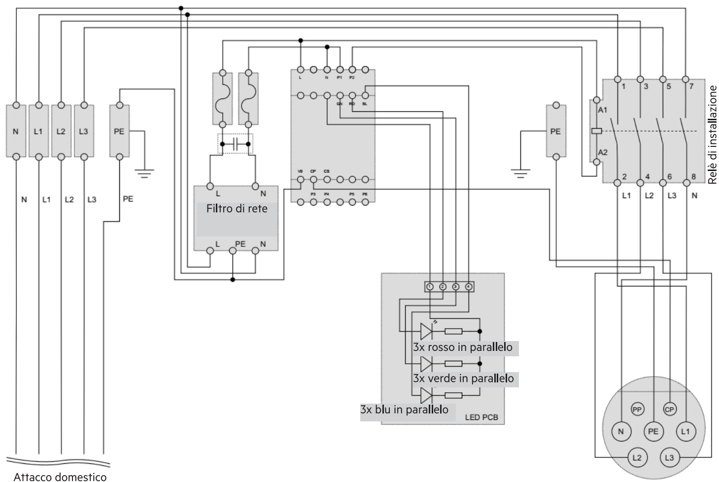
Fig. 4: Schema elettrico 11201, 11203
