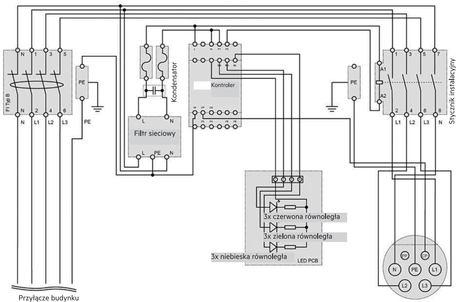
Rys. 5: Schemat połączeń 11202, 11204
