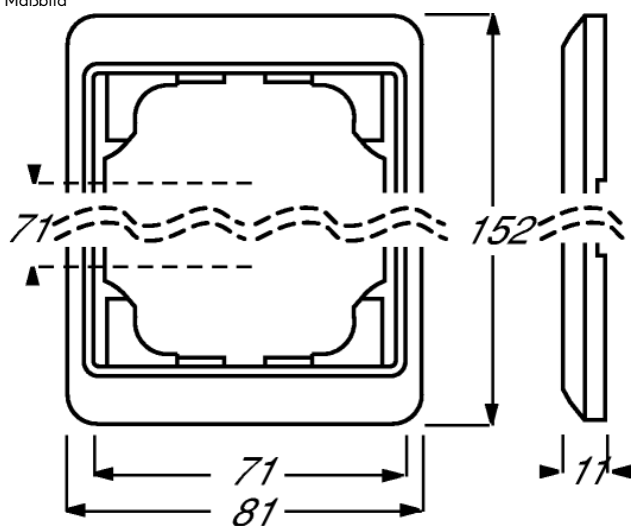
Maßbild
