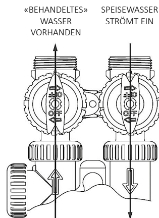
NORMALBETRIEB
