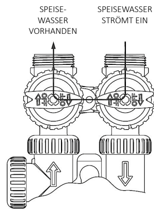
BYPASS-BETRIEB
