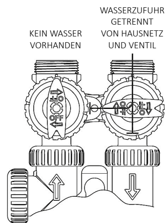
AUSSCHALT-MODUS
