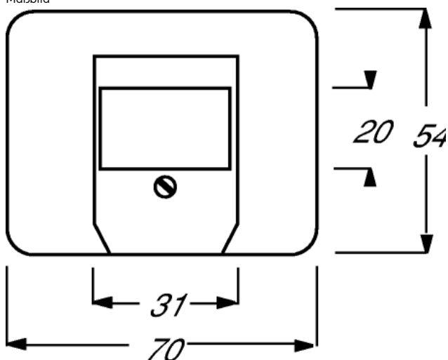
Maßbild
