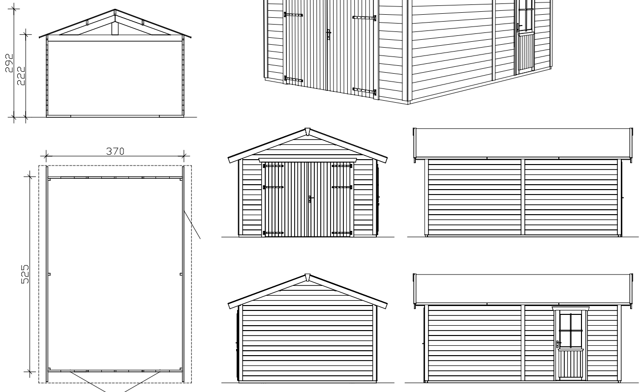
Grundriss, Schnitt und Ansichten M 1:100
