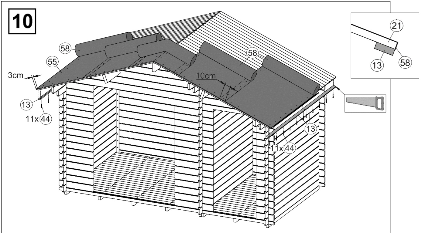
Abbildung Art.-Nr.: 253.3720.10
