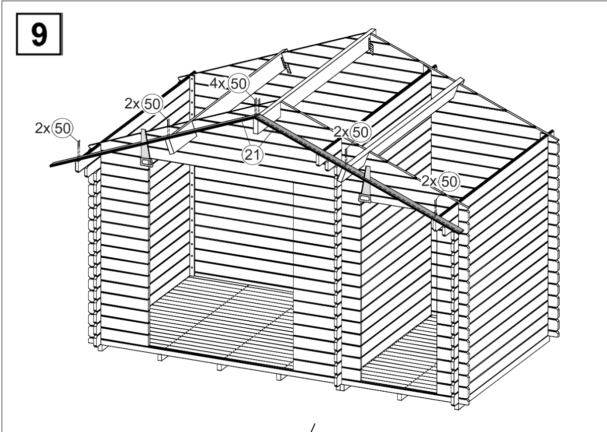
Abbildung Art.-Nr.: 253.3720.10
