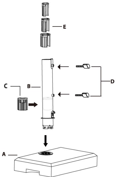
Étape 1 : Montage.
