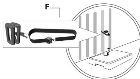
Schritt 3: Montage.
