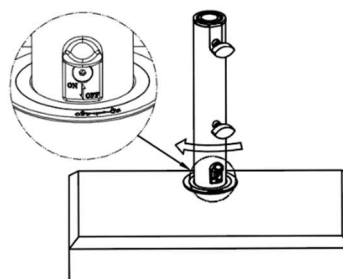
Schritt 2: Montage.
