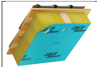
Abb. 2: Fehlstellen überkleben
