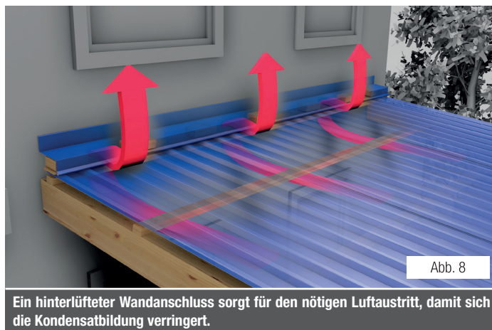
Wandanschluss mit Entlüftungsschlitzen
