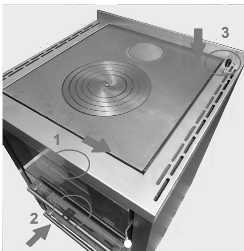
Fig. 10 - Register geschlossen
