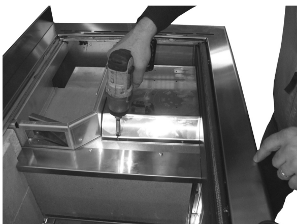
Fig. 21 - Die Schrauben entfernen
