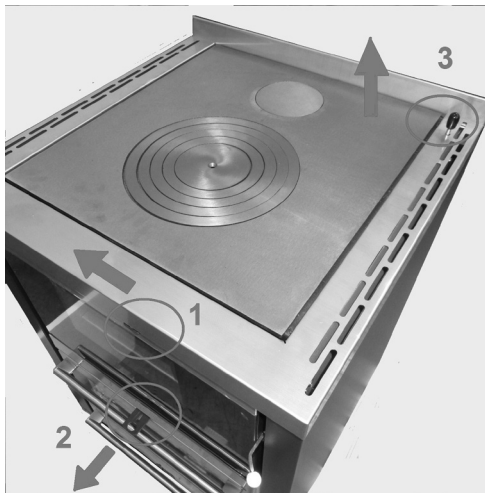
Fig. 8 - Register öffnen
