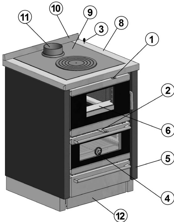
Fig. 4 - Kook 60 4.0 - Kook 70 4.0
