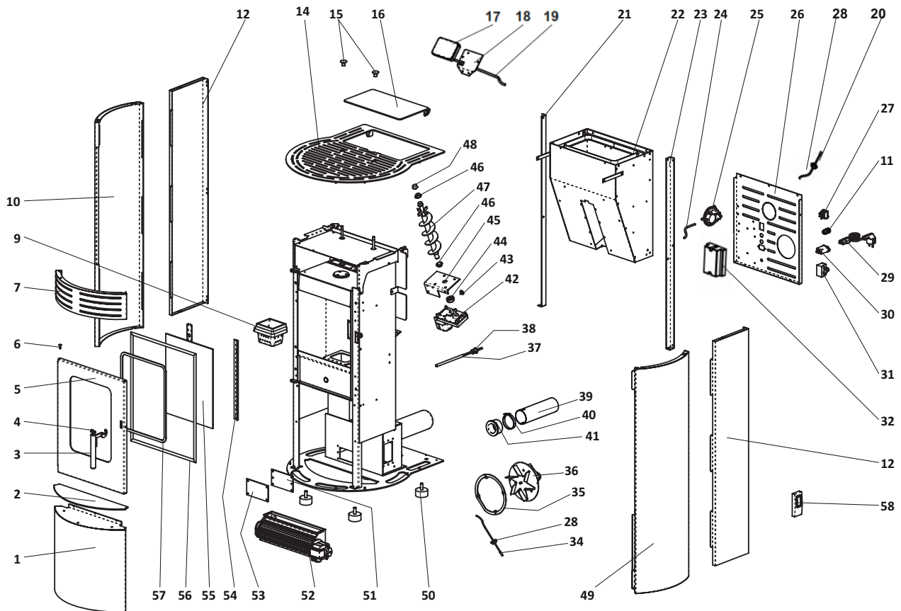
Abb. 14 Explosionszeichnung
