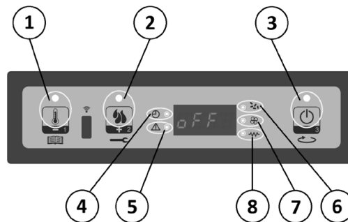
Fig. 6 - Display: Leds eingeschaltet
