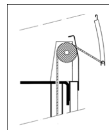
Skizze Schnurführung Section string guiding Dessin passage de la ficelle
