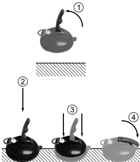
Bild 2: Montage
