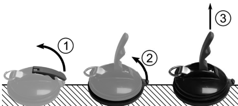
Figure 3 : détachement
