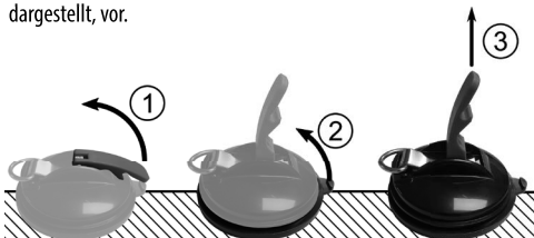
Bild 3: Lösen
