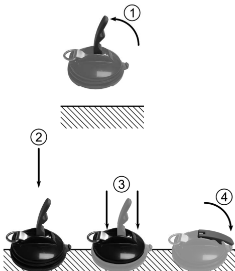
Afb. 2: Montage
