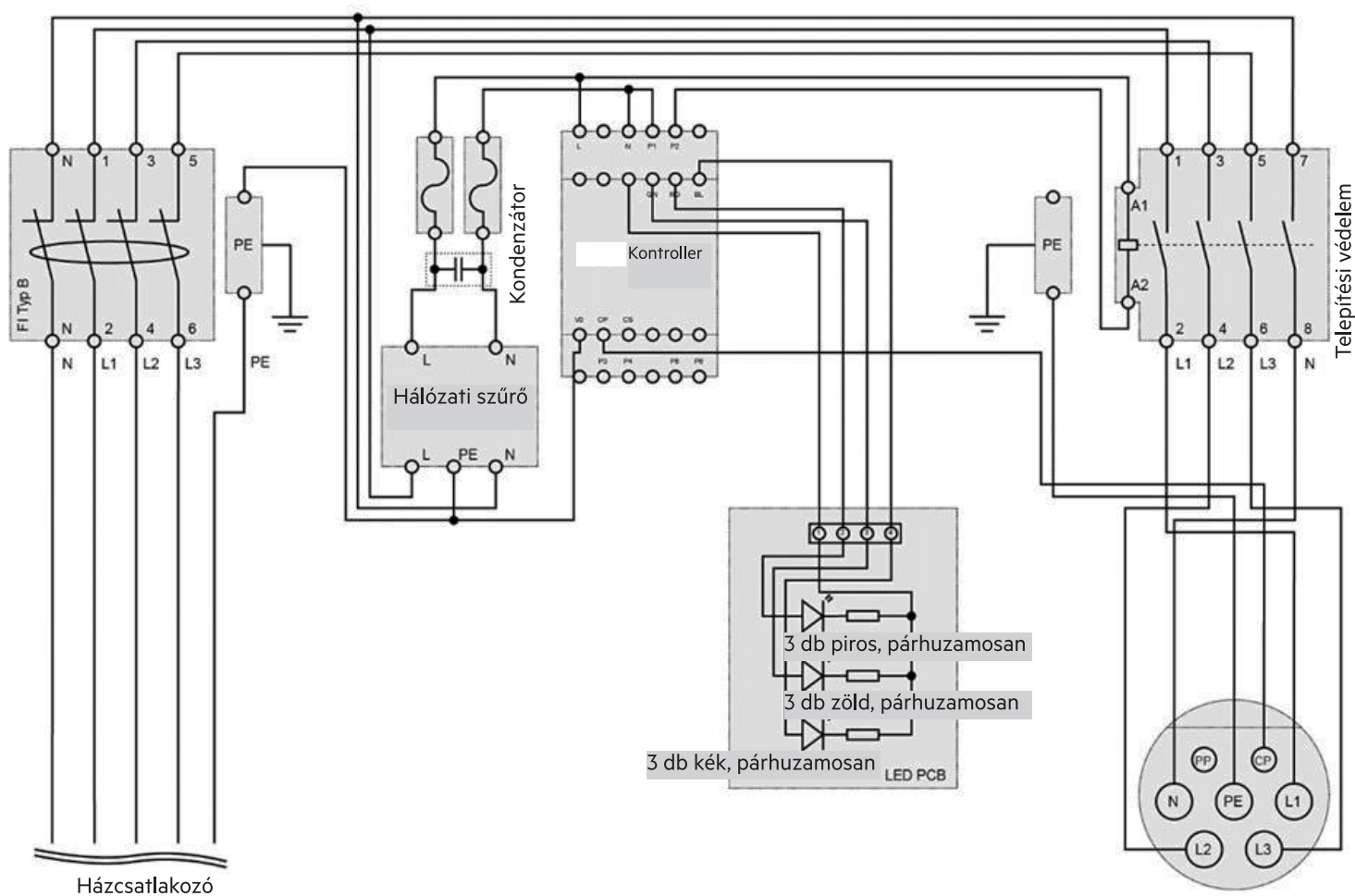
5. ábra: Kapcsolási rajz 11202, 11204
