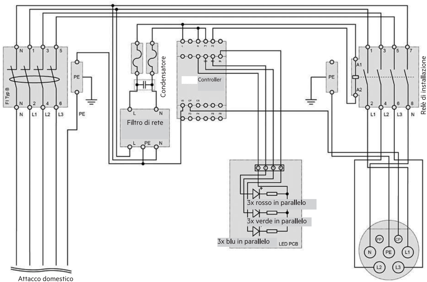
Fig. 5: Schema elettrico 11202, 11204
