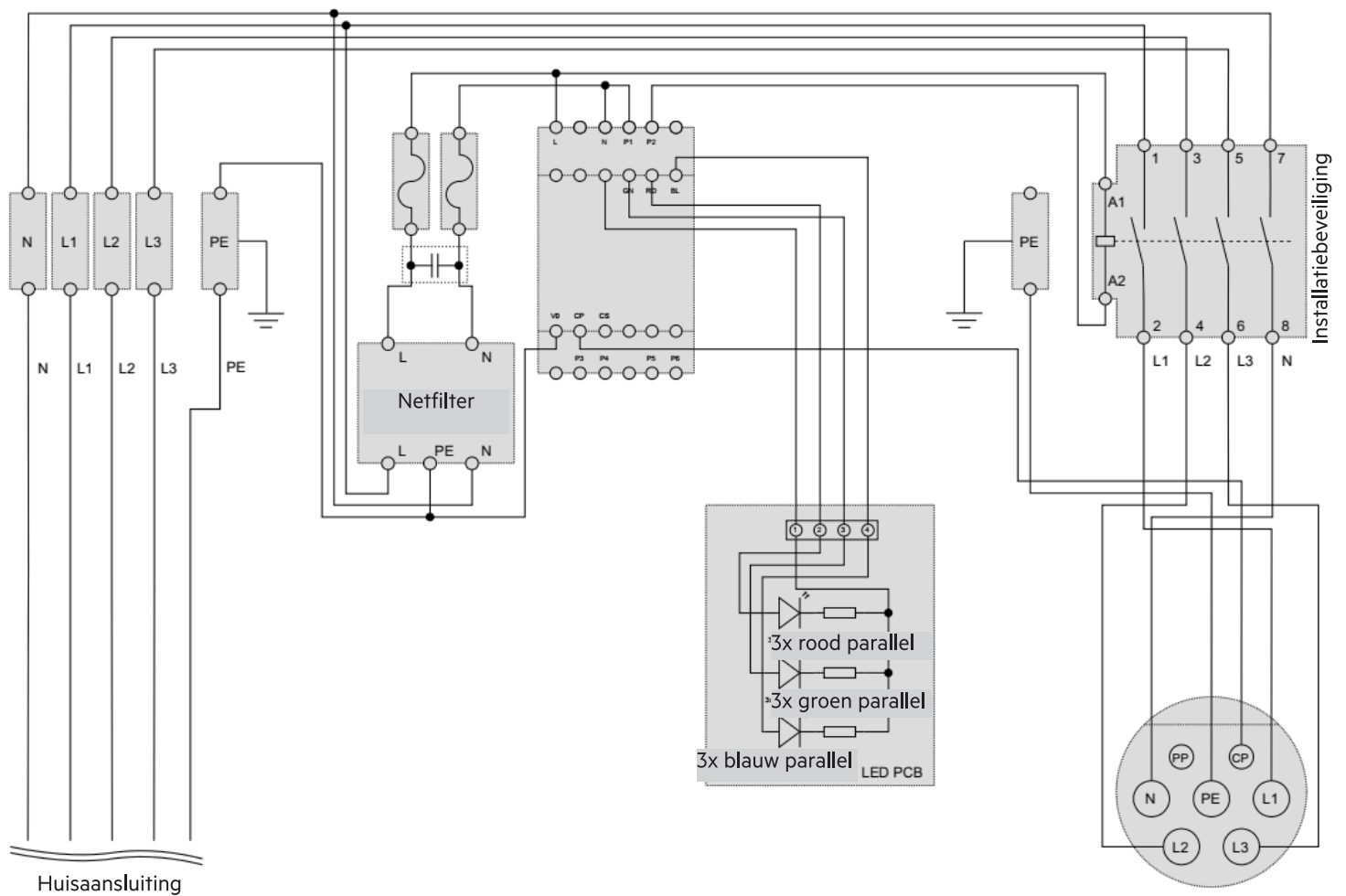
Afb. 4: Schakelschema 11201, 11203
