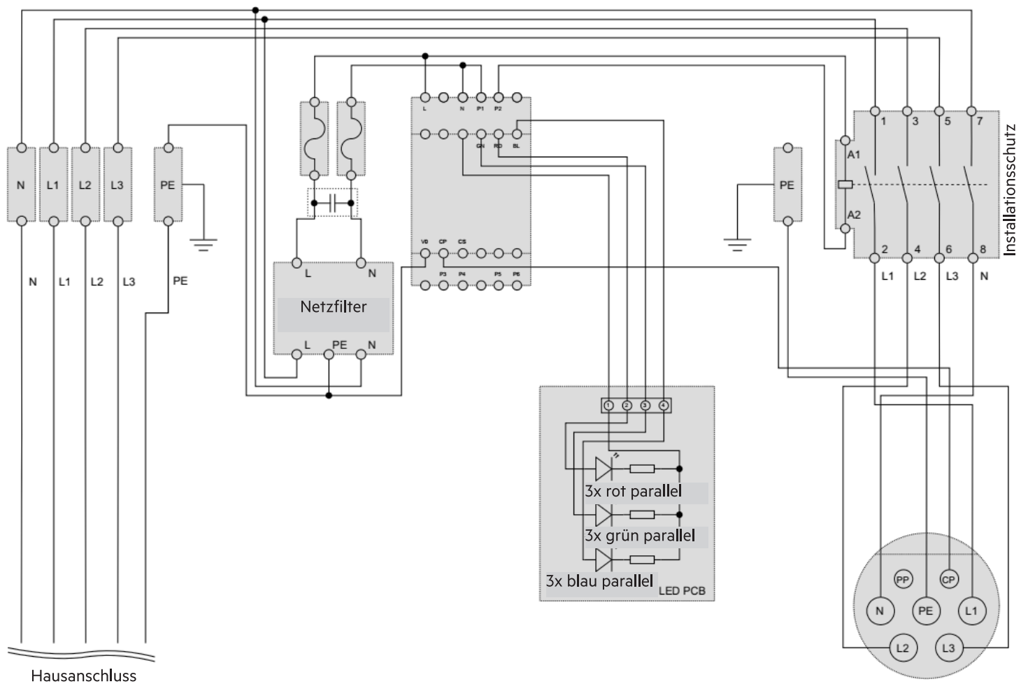
Abb. 4: Schaltplan 11201, 11203
