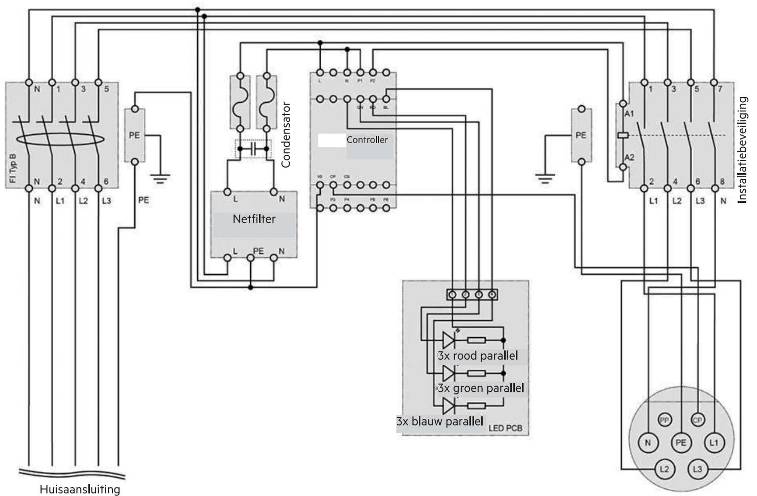
Afb. 5: Schakelschema 11202, 11204
