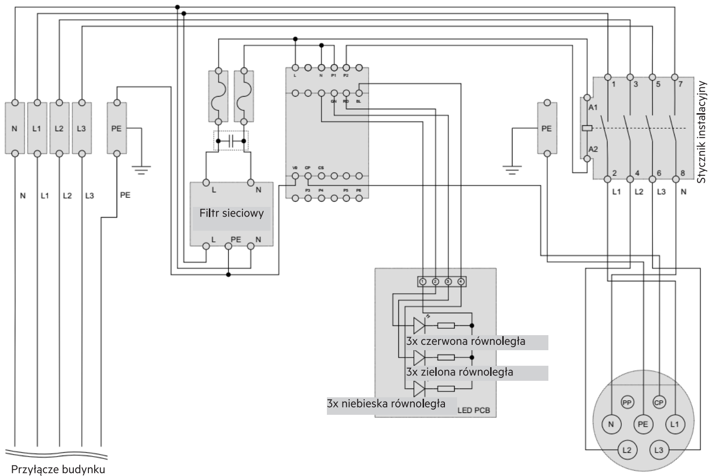
Rys. 4: Schemat połączeń 11201, 11203
