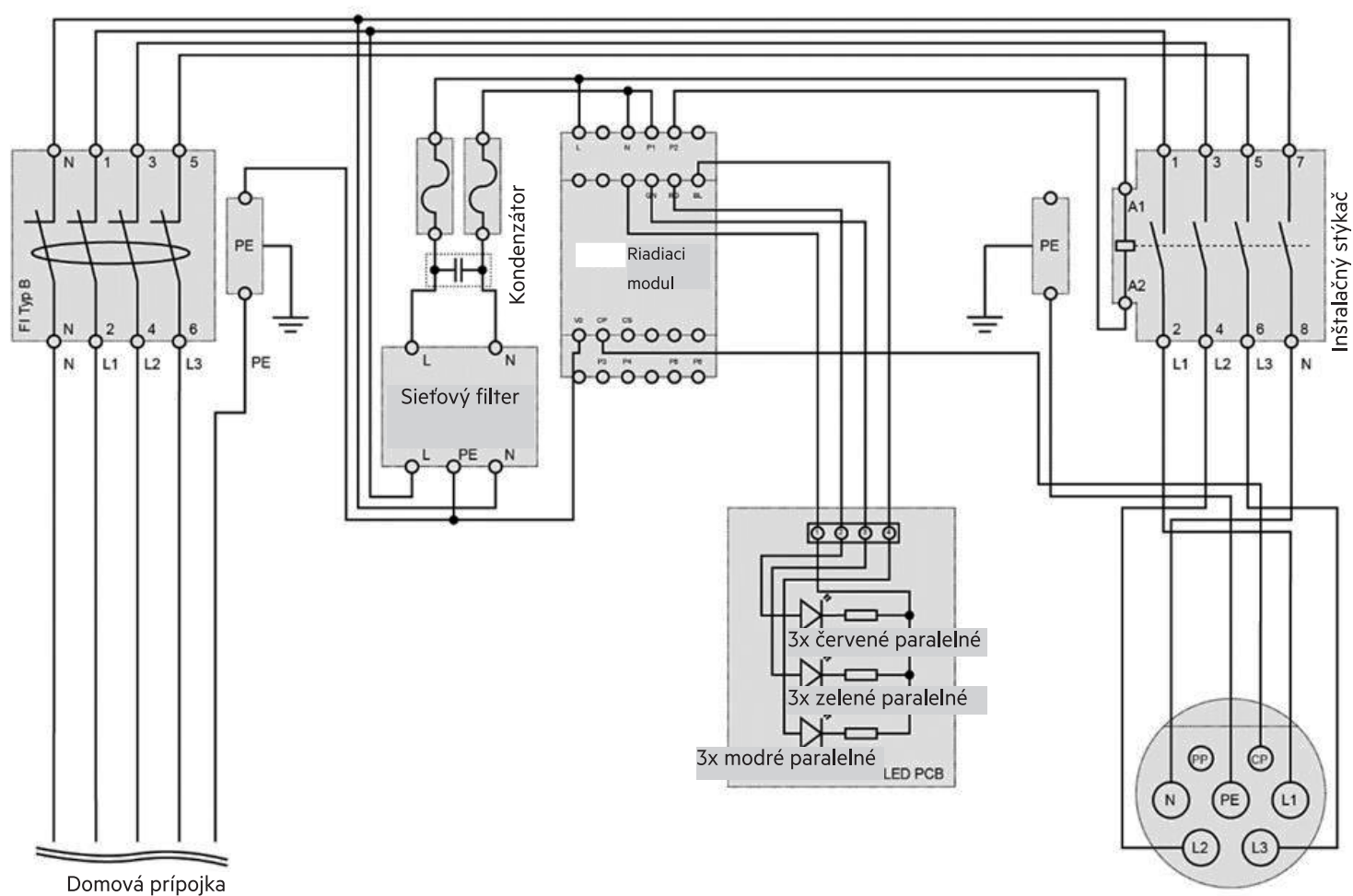
Obr. 5: Schéma zapojenia 11202, 11204
