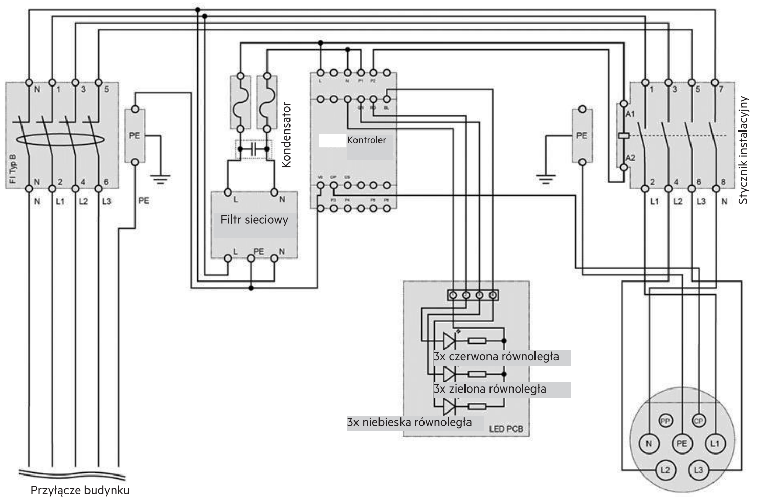
Rys. 5: Schemat połączeń 11202, 11204
