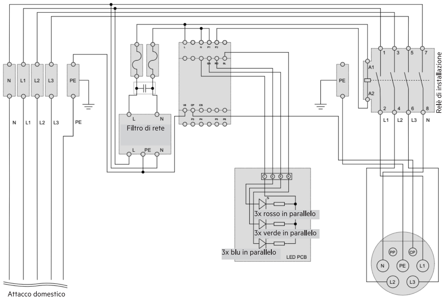
Fig. 4: Schema elettrico 11201, 11203
