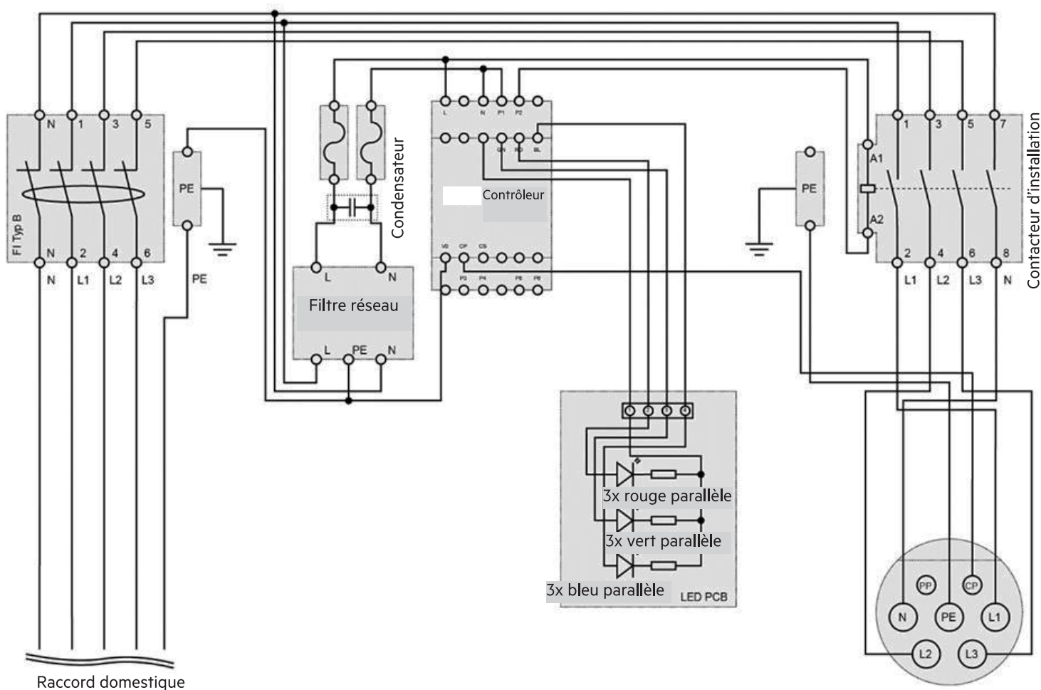
Fig. 5 : Schéma de câblage 11202, 11204
