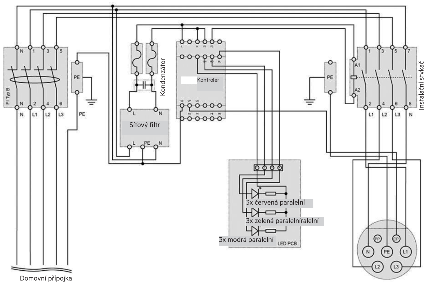
Obr. 5: Schéma zapojení: 11202, 11204
