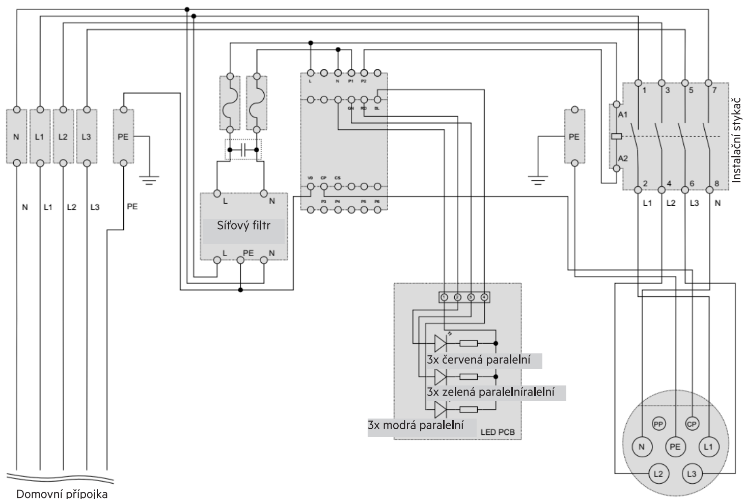
Obr. 4: Schéma zapojení 11201, 11203
