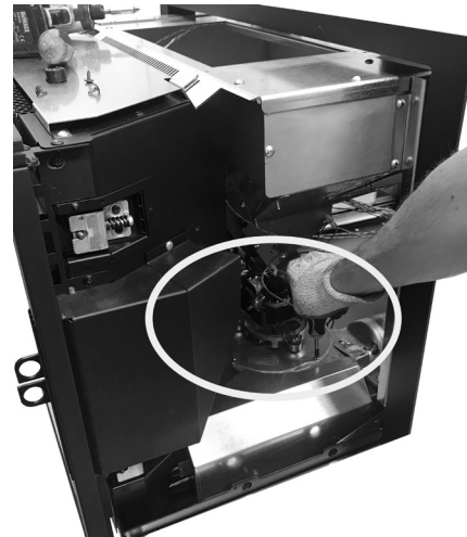
Fig. 71 - Die Schrauben entfernen.
