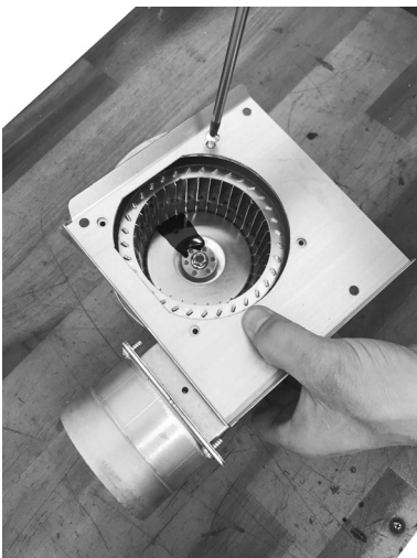
Fig. 33 - Den Deckel fixieren.
