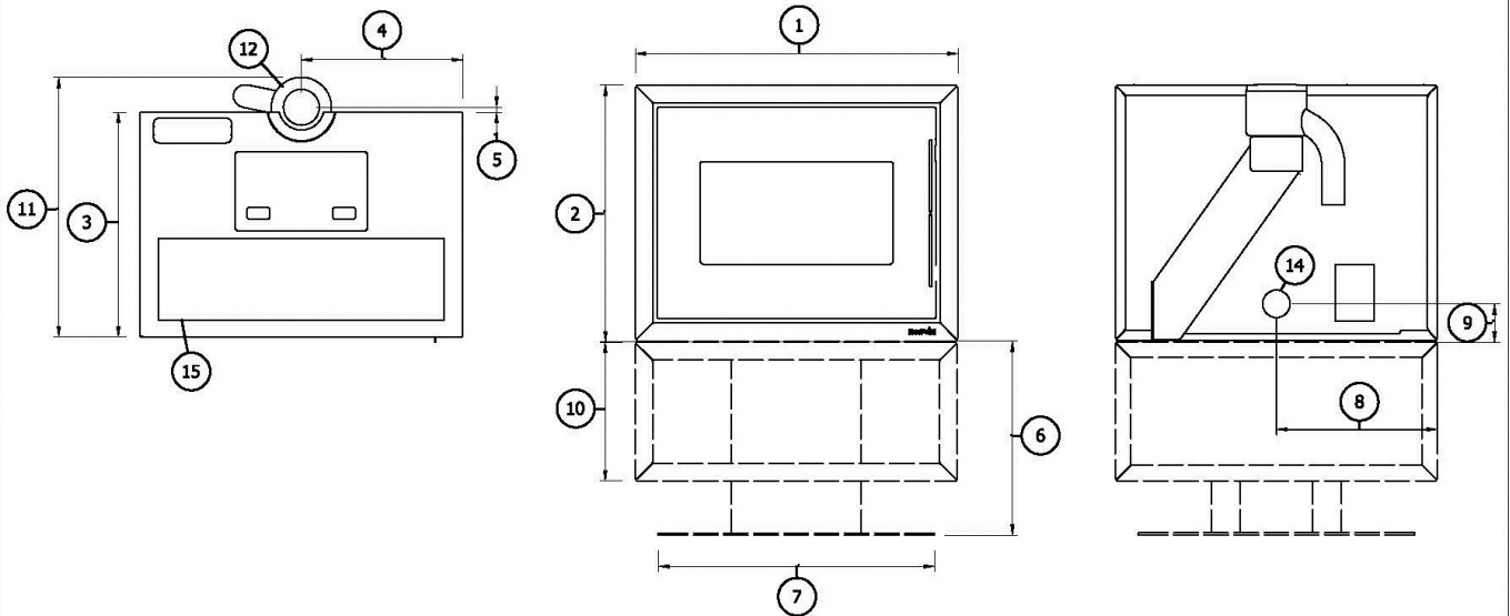
Fig. 14 - Allgemeine Abmessungen: MODO AIRTIGHT
