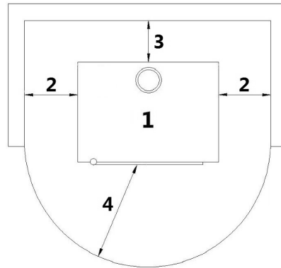
Fig. 15 - Allgemeine Installation
