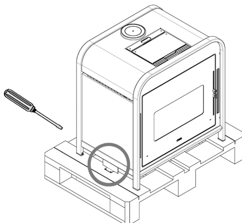
Fig. 1 - Lösen Schrauben + Bügel
