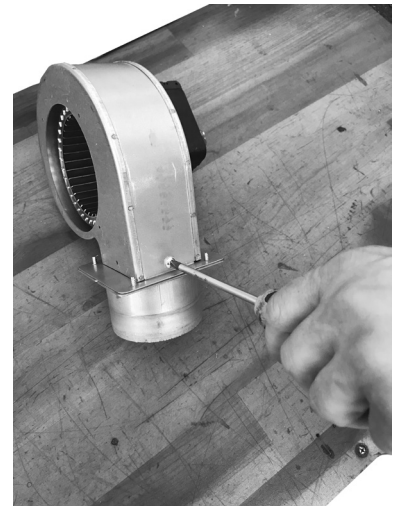
Fig. 32 - Mit Schrauben fixieren.
