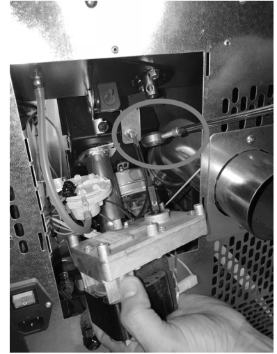
Fig. 64 - Getriebemotor entfernen
