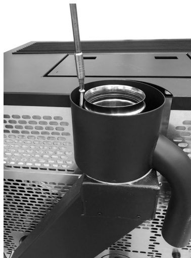
Fig. 58 - konzentrische Rohr befestigen
