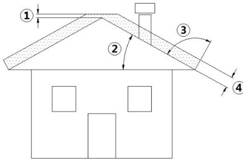
Fig. 3 - Geneigtes Dach
