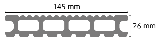
Kovalex® Exklusiv Hohlkammerprofil (Länge: 1 m - 6 m*)
