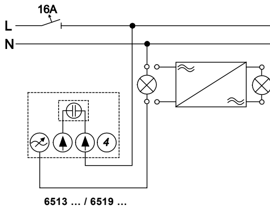
Abb. 2: Dimmerbetrieb
