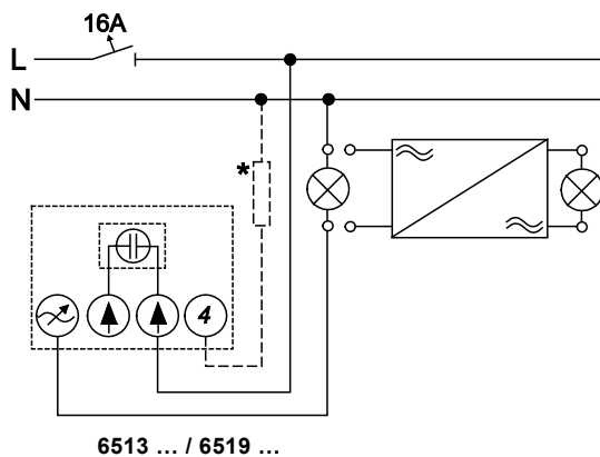
Abb. 4: Dimmerbetrieb mit Spannungssensor
