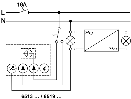
Abb. 3: Dimmer in Wechselschaltung
