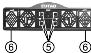
Figura 6: Montaggio targa
