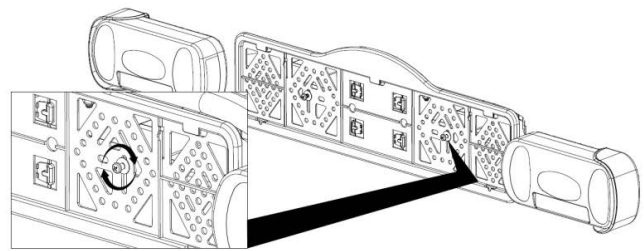
Figura 5: Montaggio portatarga
