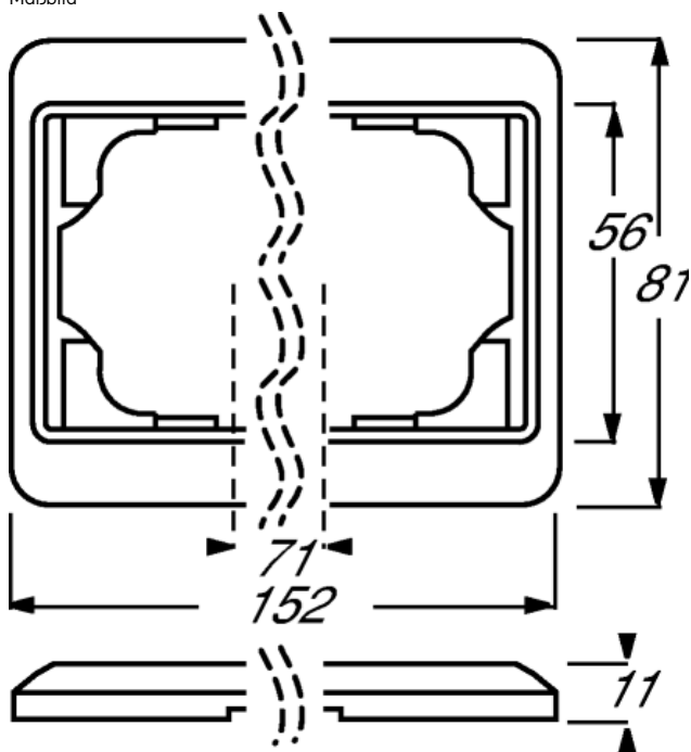
Maßbild
