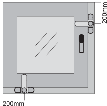
Abbildung 2: Empfohlene Montageposition
