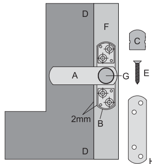
Abbildung 3: Montage des Befestigungsblocks
