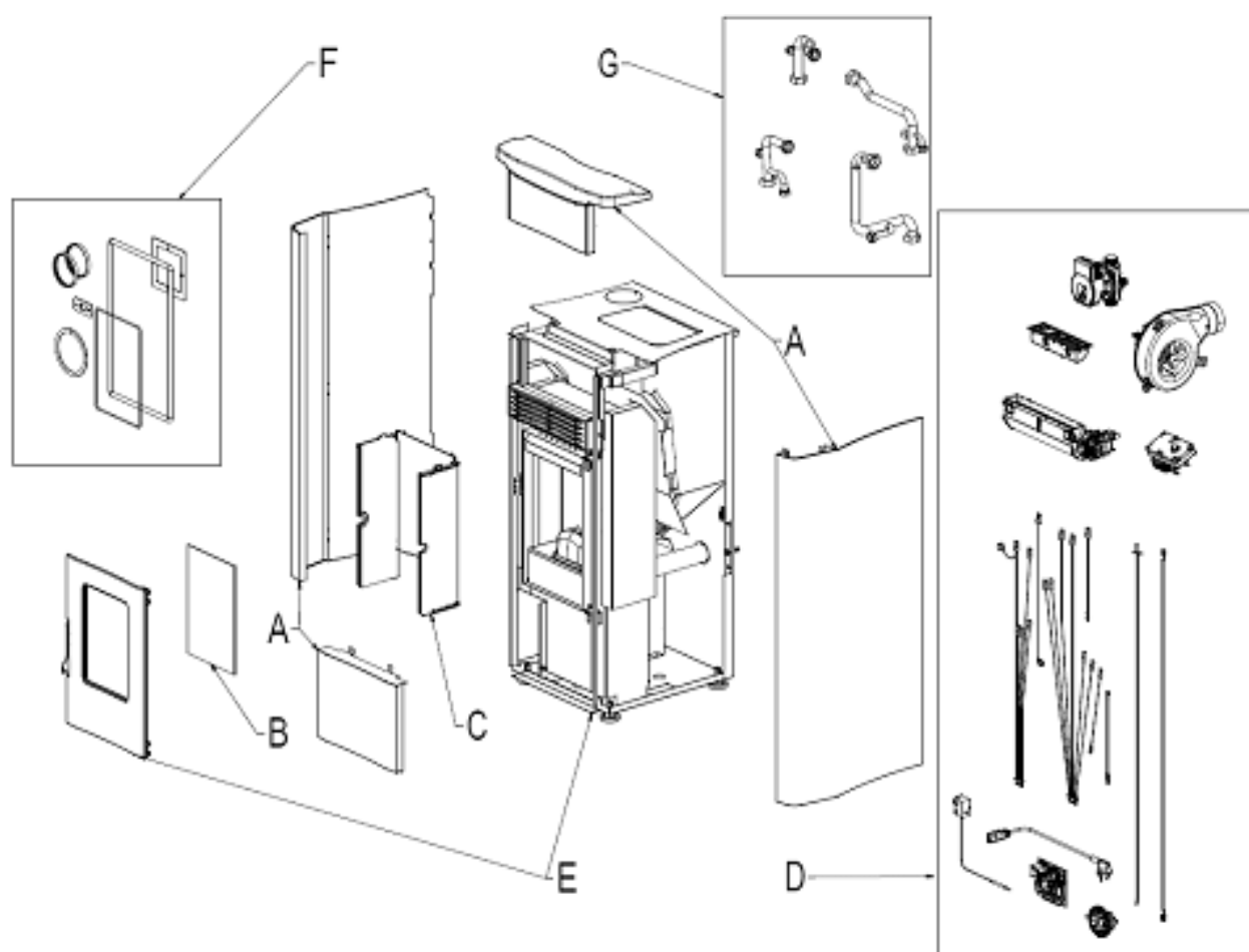
Fig. 1 - Explosionszeichnung
