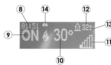
Fig. 9 - Display
