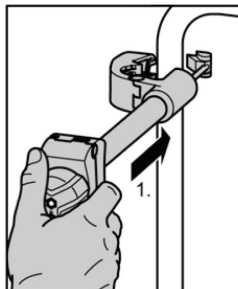
Bild 9: Rahmenhalter ansetzen
