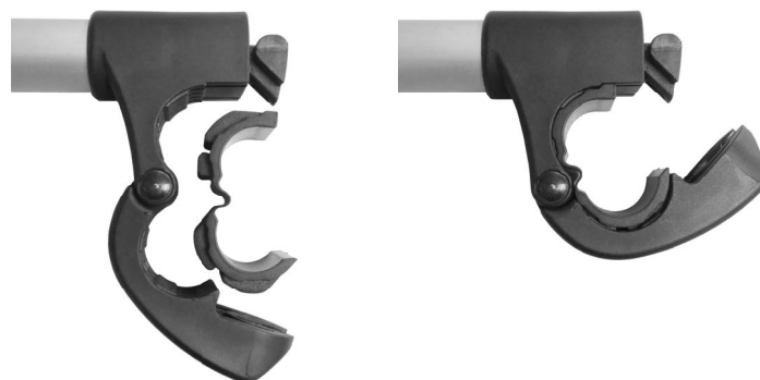
Bild 8: Einsetzen des Reduzierstücks
