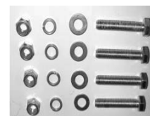
4 x Schraube M8 x 50 4 x Scheibe 8 mm 4 x Federring 4 x Mutter M8
