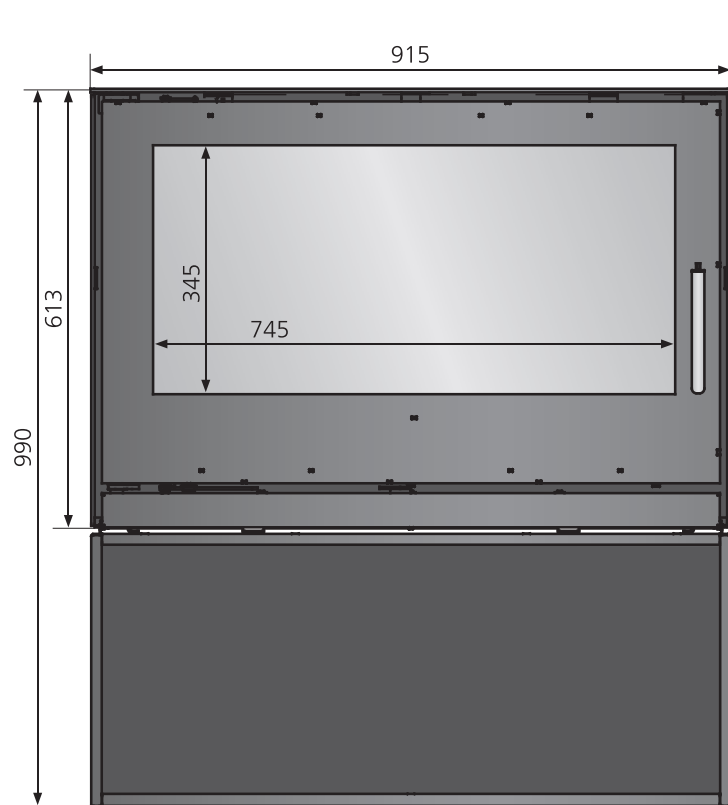
MZ Dias XL mit Box
