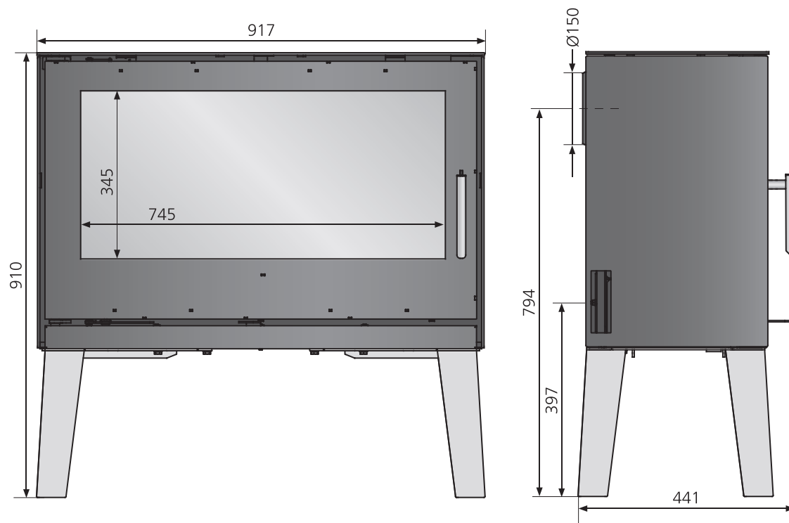
MZ Dias XL mit Holzfußset
