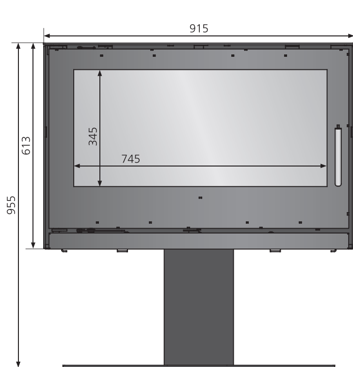
MZ Dias XL mit Standfuss
