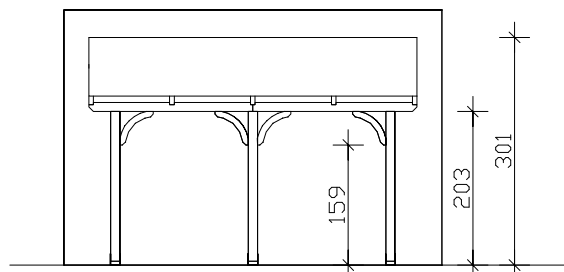
Frontansicht
