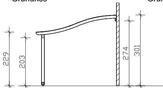
Seitenansicht
