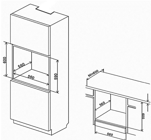
Einbauskizze
