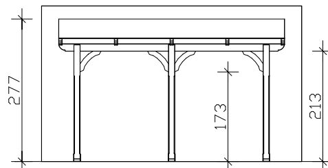
Frontansicht
