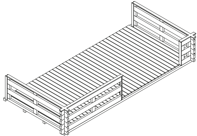
Grundriss, Schnitt und Ansichten M 1:100
