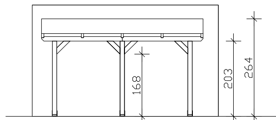
Frontansicht
