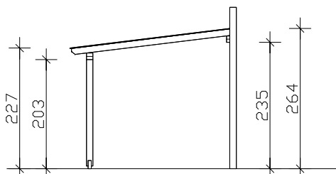
Seitenansicht
