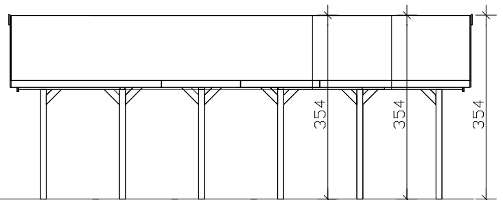
Seitenansicht
