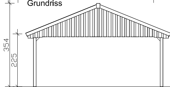
Vorderansicht
