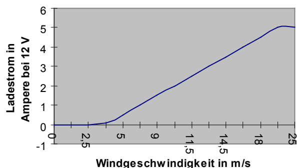
Leistungskurve WG 504
