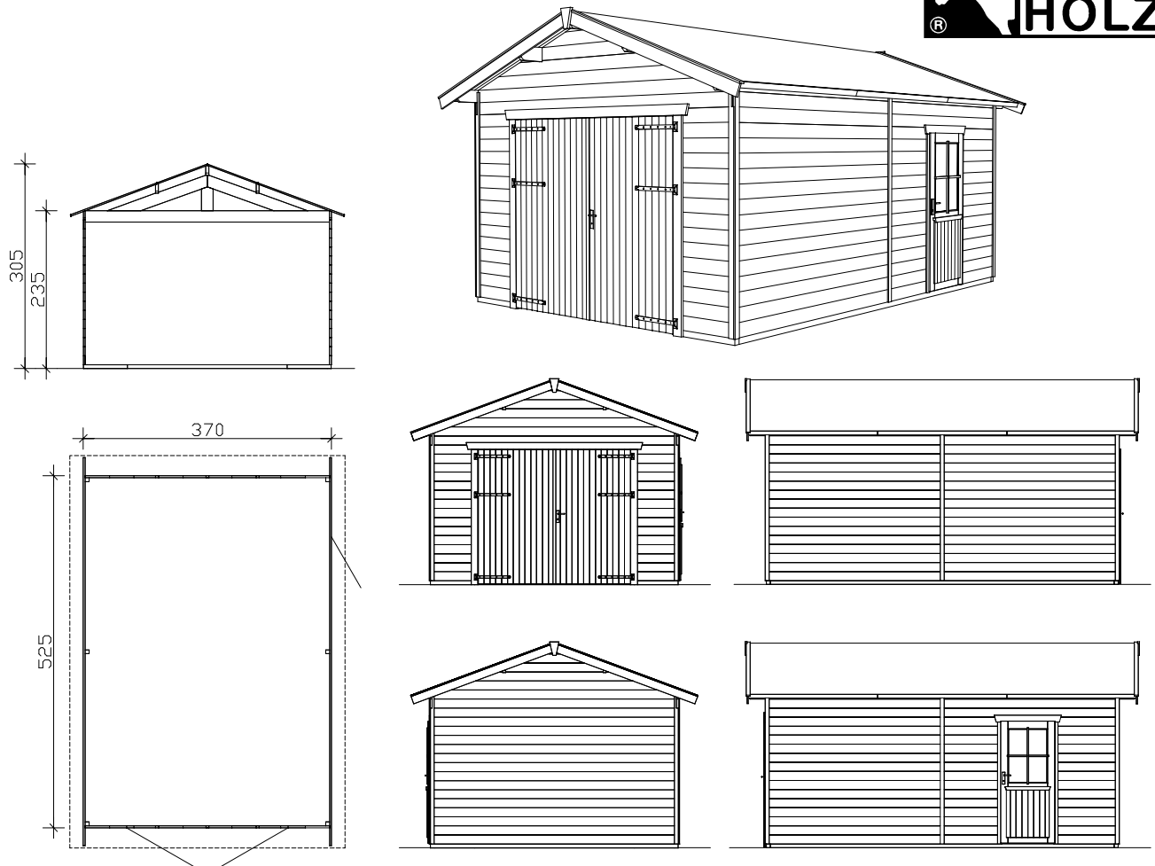
Grundriss, Schnitt und Ansichten M 1:100
