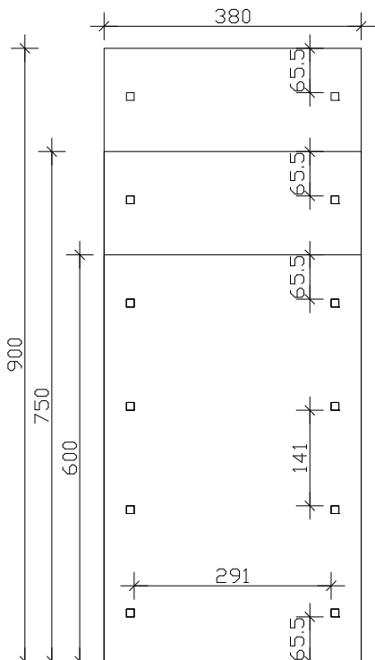
Grundriss
