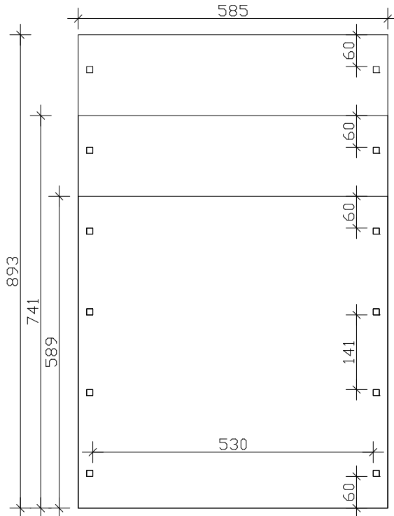
Grundriss
