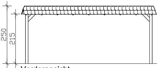
Vorderansicht
