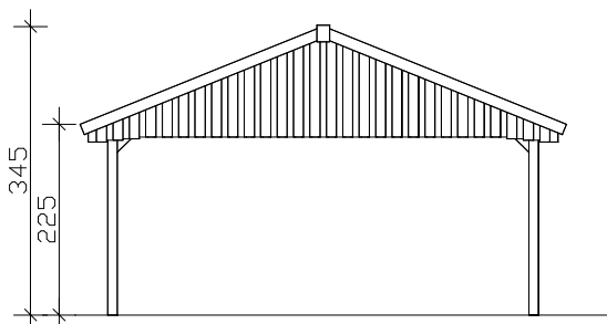
Vorderansicht
