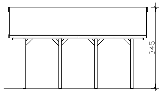
Seitenansicht
