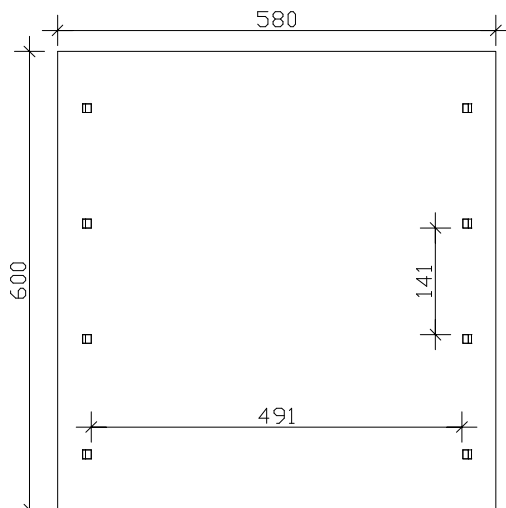
Grundriss
