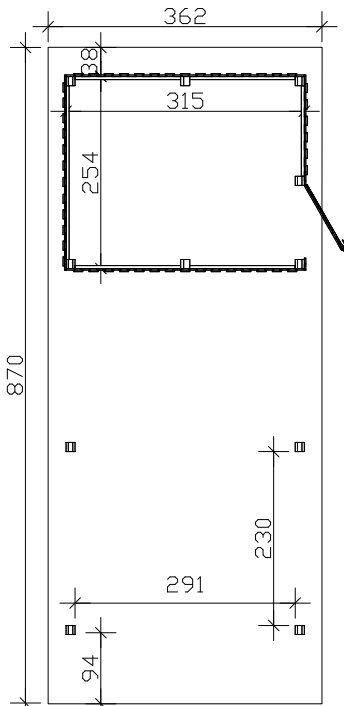
Grundriss
